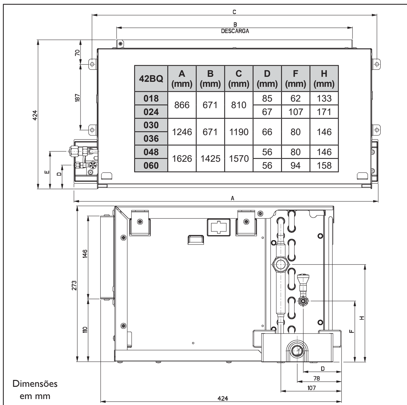
FIG. 17 - DIMENSIONAL 42BQ
